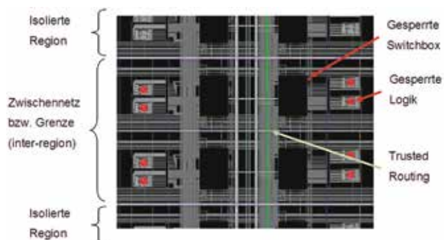
Bild 5: Spezielles Bussystem, das an definierte Switchboxen angeschlossen ist.
