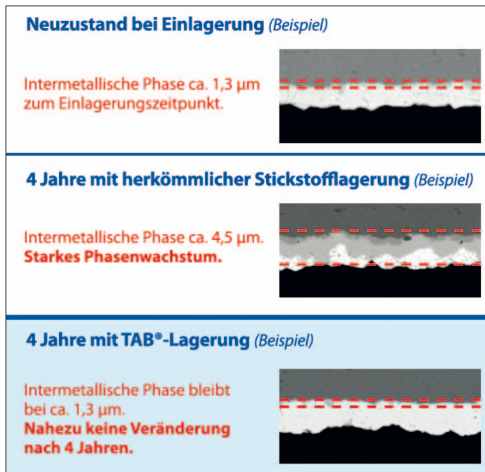
Bild 16: Bei der Lagerung nach TAB ist nahezu kein intermetallisches Phasenwachstum feststellbar
