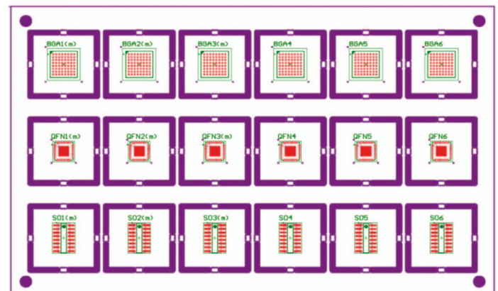
Bild 1: Test-LP mit Sub-Leiterplatten zum leichten Heraustrennen einzelner Regionen
